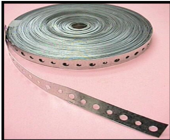
▲ 33000 - Pipe Hang- er Strap- 100' per Roll
